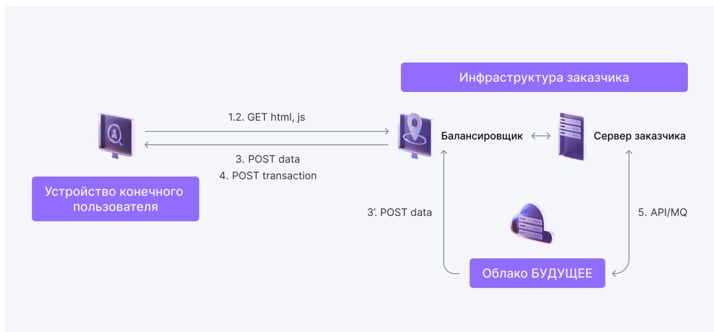
Рисунок 4. Схема передачи контрольных данных через ИТ-инфраструктуру Заказчика.
